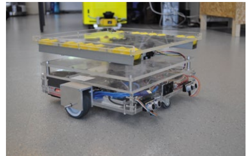
Modellfahrzeug zur Datensynthese kostengünstiger Sensoren. Quelle: Maximilian Zwingel
